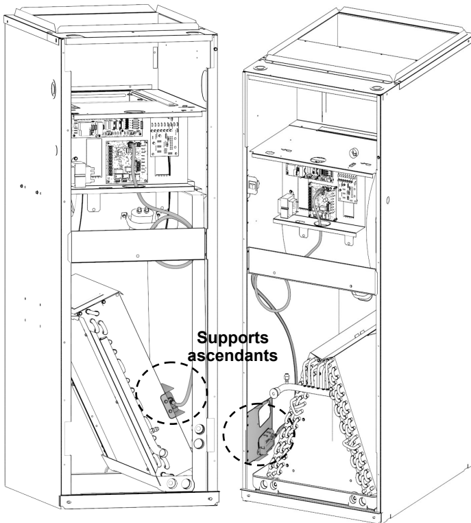
Modèles à serpentín incliné
