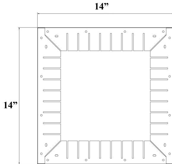
Figure 6 : Dimensions du connecteur de gaine
