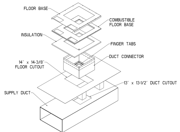
Figure 7 : Installation typique du connecteur de gaine
