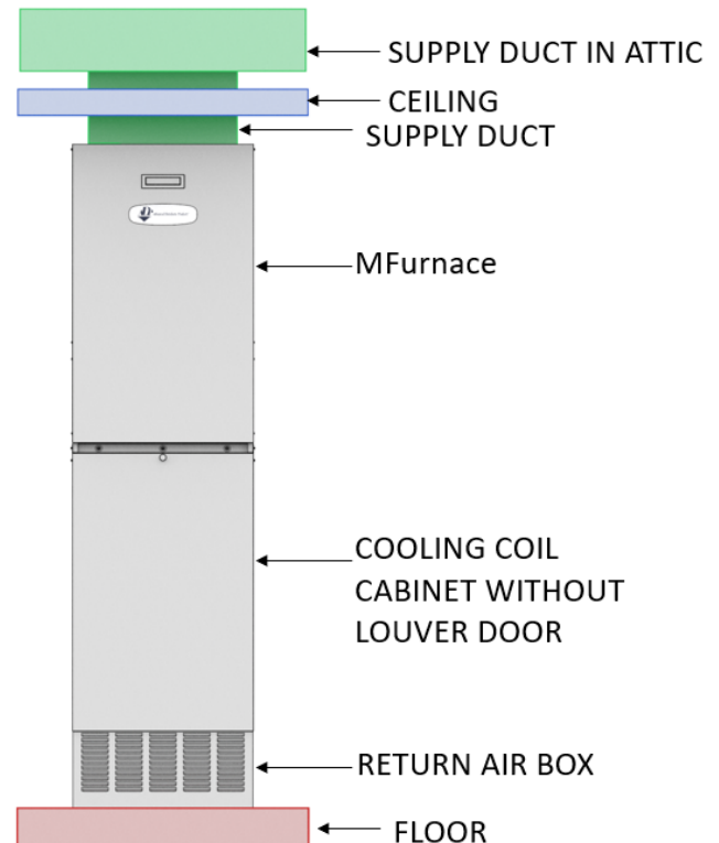
Figure 10 : Installation ascendante typique avec conduit d'alimentation et boîte de retour d'air
