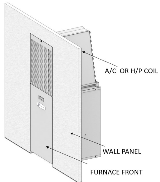
Figure 3 : Exemple d'installation d'une alcôve
